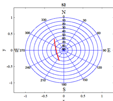
شکل 13: مشاهدات سمت-ارتفاع ماهواره از دید حسگر S_2 .
