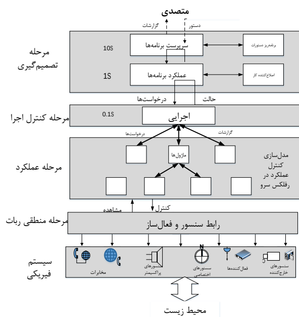
شکل 24. معماری LAAS
