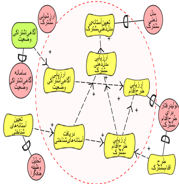
شکل شماره ۸. نمودار هدف‌ها برای نقش‌پیشه تولید رفتار برای طرح اقدام مشترک
