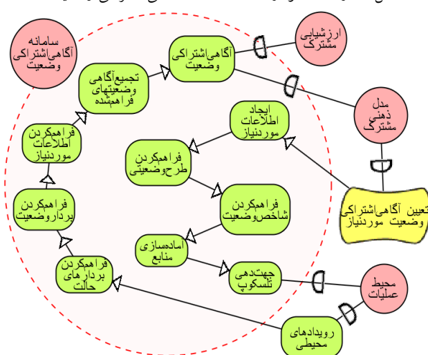
شکل شماره ۱۱. نمودار هدف‌ها سامانه آگاهی اشتراکی وضعیت
