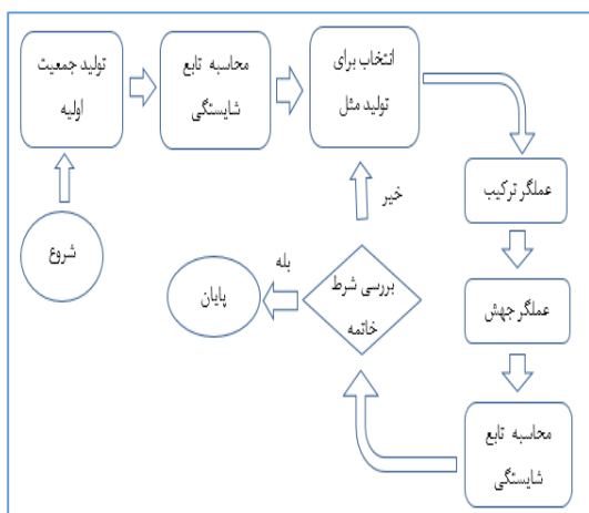
شکل 3: فلوچارت الگوریتم ژنتیک
