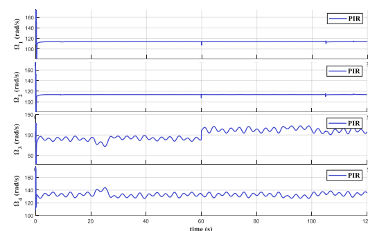
شکل ۳۳. سرعت چرخش روتورها برای سناریو سوم.
