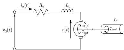
شکل ۲. دیاگرام مداری موتور بدون جاروبک.
