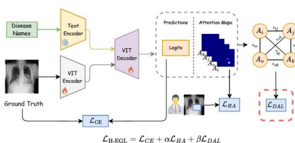
شکل ۱. چارچوب یادگیری هدایت‌شده با تبیین ترکیبی روش H-EGL [۵].
