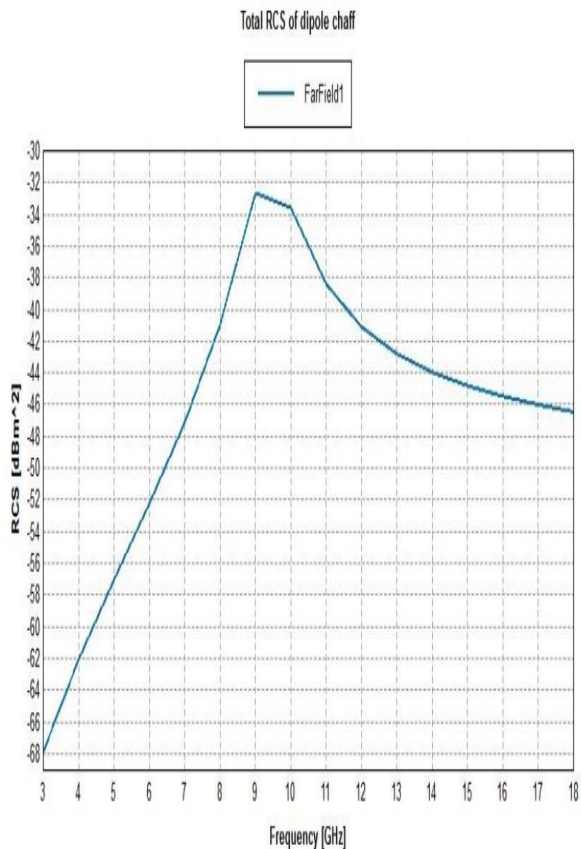
شکل ۹. سطح مقطع و پهنای باند مؤثر راداری دوقطبی چف
