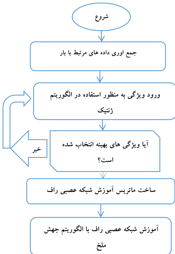
شکل ۱: فلوچارت پیشنهادی انتخاب ویژگی های بهینه با الگوریتم ژنتیک به منظور استخراج ویژگی های بهینه و ویژگی هایی که بیشترین تاثیر را در پیش بار دارند از مقاله [۲۳]
