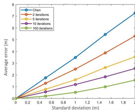
شکل ۶: خطای تخمین روش‌های Chan و I-Chan2 بر اساس تعداد
