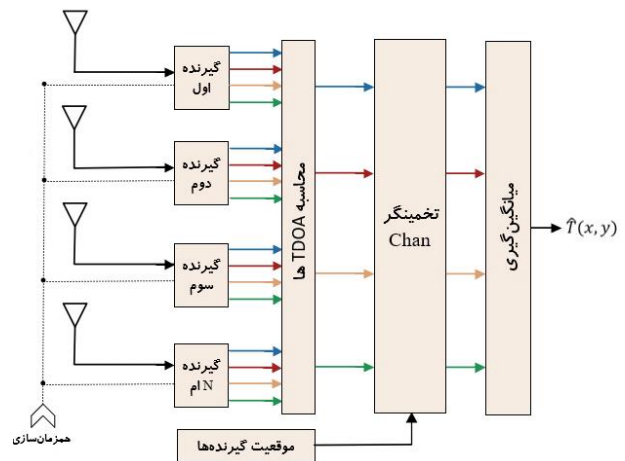
شکل ۲. نمودار بلوکی روش I-Chan برای ۴ تکرار نمونه‌برداری
