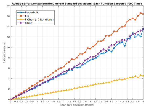
شکل ۵. مقایسه خطای ۴ روش در حضور نویز متفاوت
