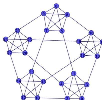
شکل ۱۶. گراف سرپینسکی S_5^2 ایجاد شده با نرم‌افزار گفی
