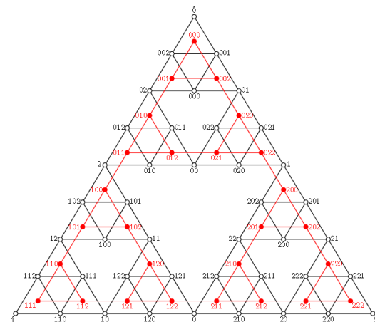
شکل ۱۹. مقایسه هم‌بندی دو گراف \hat{S}_3^3, S_3^3
