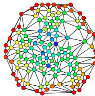
شکل ۵. شبکه دنیای کوچک
