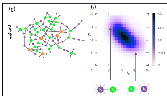
شکل ۹. شبکه‌های بی طرف، هم تیپ، ناهم تیپ
