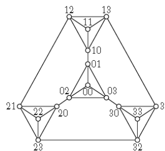
شکل ۱۵. گراف‌های سرپینسکی S_4^2
