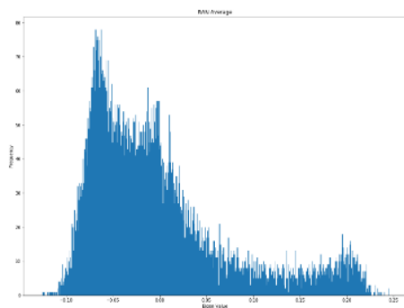
شکل ۲۹. مقادیر ویژه برای ۱۰ شبکه تصادفی آپولونین
