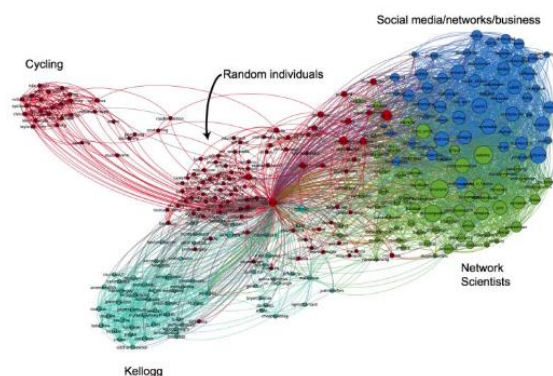
شکل ۶. شبکه مقیاس آزاد
