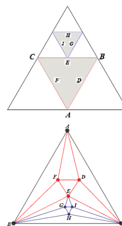
شکل ۲۲. مرحله دوم شبکه gasket (بالا) و مرحله دوم شبکه RSN (پایین)
