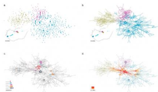
شکل ۱. نمونه‌ای از شبکه‌های پیچیده
