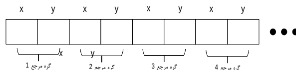
شکل 6. کروموزوم راه‌حل‌ها
