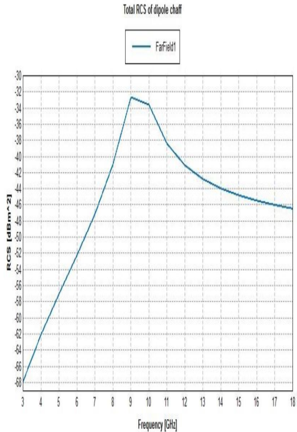
شکل ۹. سطح مقطع و پهنای باند مؤثر راداری دوقطبی چف
