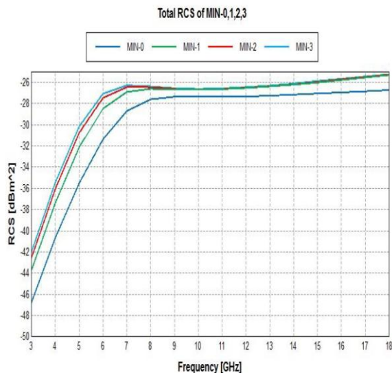
شکل ۱۱. مقایسه سطح مقطع و پهنای باند مؤثر راداری المان چف فرکتال مینکوفسکی افزایشی در مرتبه‌های صفر، یک، دو و سه
